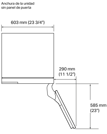
APERTURA DE PUERTA 115°
